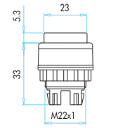
Çıkık Kafalı, Yaylı Round Button High Position
