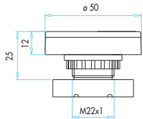
Çiftli Düz Kafalı, Yaylı Double Head
