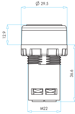
Düz Kafalı Yaylı Buton Round Push Button
